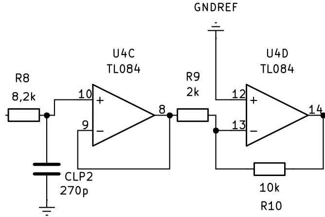
Figura 10: Pasabajos R8–CLP2, seguidor U4C y amplificador inversor U4D. El valor de R9 utilizado es 2,2 kΩ; el rótulo de 2 kΩ del esquema no corresponde al valor montado.
